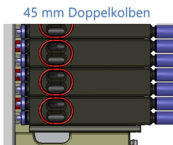
Beispiel einer Hybrid-Lösung links 45er Büchsen – rechts 90er NI-Büchsen
